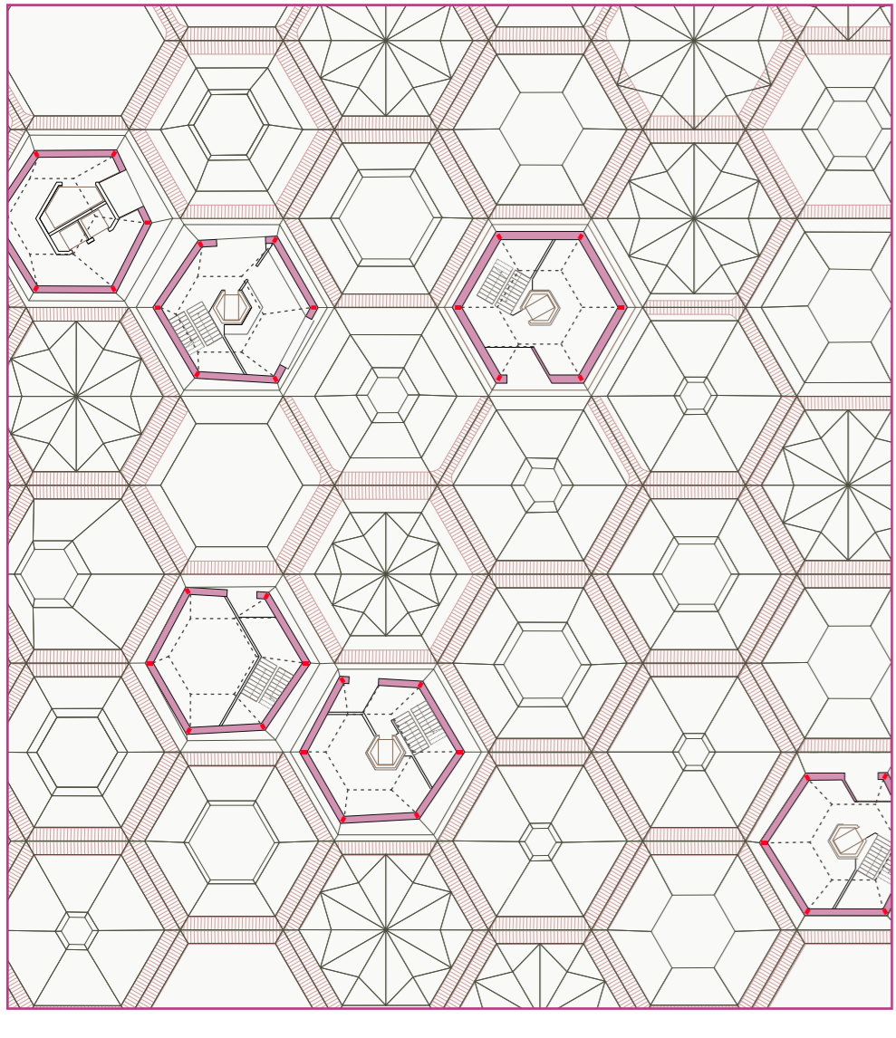
rehearsal studio level (+12,50m.) 中排演室
